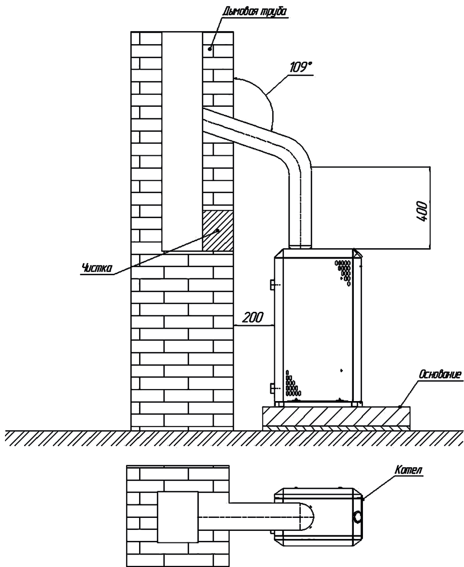
Рисунок 1. Схема размещения котлов
